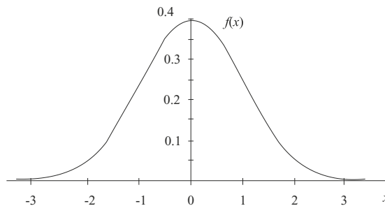
Figura 5.5. Gráfica de la función de densidad f(x) de (5.6) (Elaborada por los autores con el software libre R)
