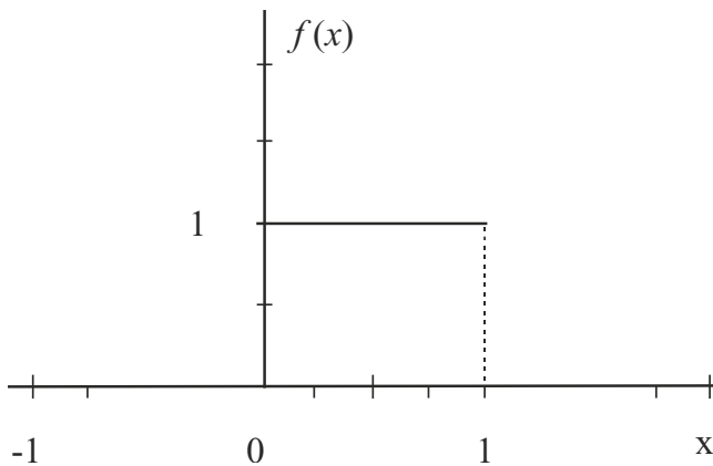
Figura 5.6. Gráfica de la función de densidad f(x) de (5.7) (Elaborada por los autores con el software libre R)
